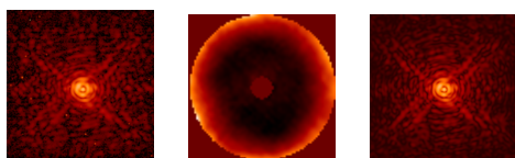
FIG. 3 – Reconstruction de défocus à partir de données acquises sur SPHERE. De gauche à droite : image coronagraphique acquise sur le détecteur, aberrations reconstruites par COFFEE dans la pupille d'entrée du système, image calculée par COFFEE à partir des aberrations estimées.
