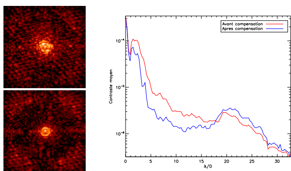
FIG. 4 – Optimisation du contraste sur l'instrument SPHERE. A gauche : images expérimentales acquises via le détecteur scientifique avant (haut) et après (bas) compensation des aberrations \phi_u . A droite : tracé de l'intensité moyenne circulaire normalisée avant (rouge) et après (bleu) compensation (1 : pas de coronagraphe) calculée à partir des deux images de gauche.
