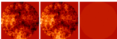
FIG. 2 – Performances de COFFEE : simulation. De gauche à droite : aberrations \phi_u simulées, aberrations \hat{\phi}_u estimées par COFFEE, différence absolue |\phi_u - \hat{\phi}_u| .
